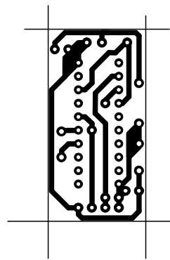
Lötseite
