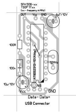
Bestückungsseite
